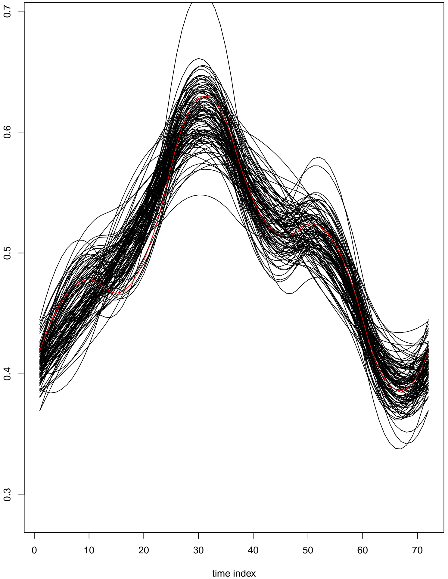
posterior samples of lambda
