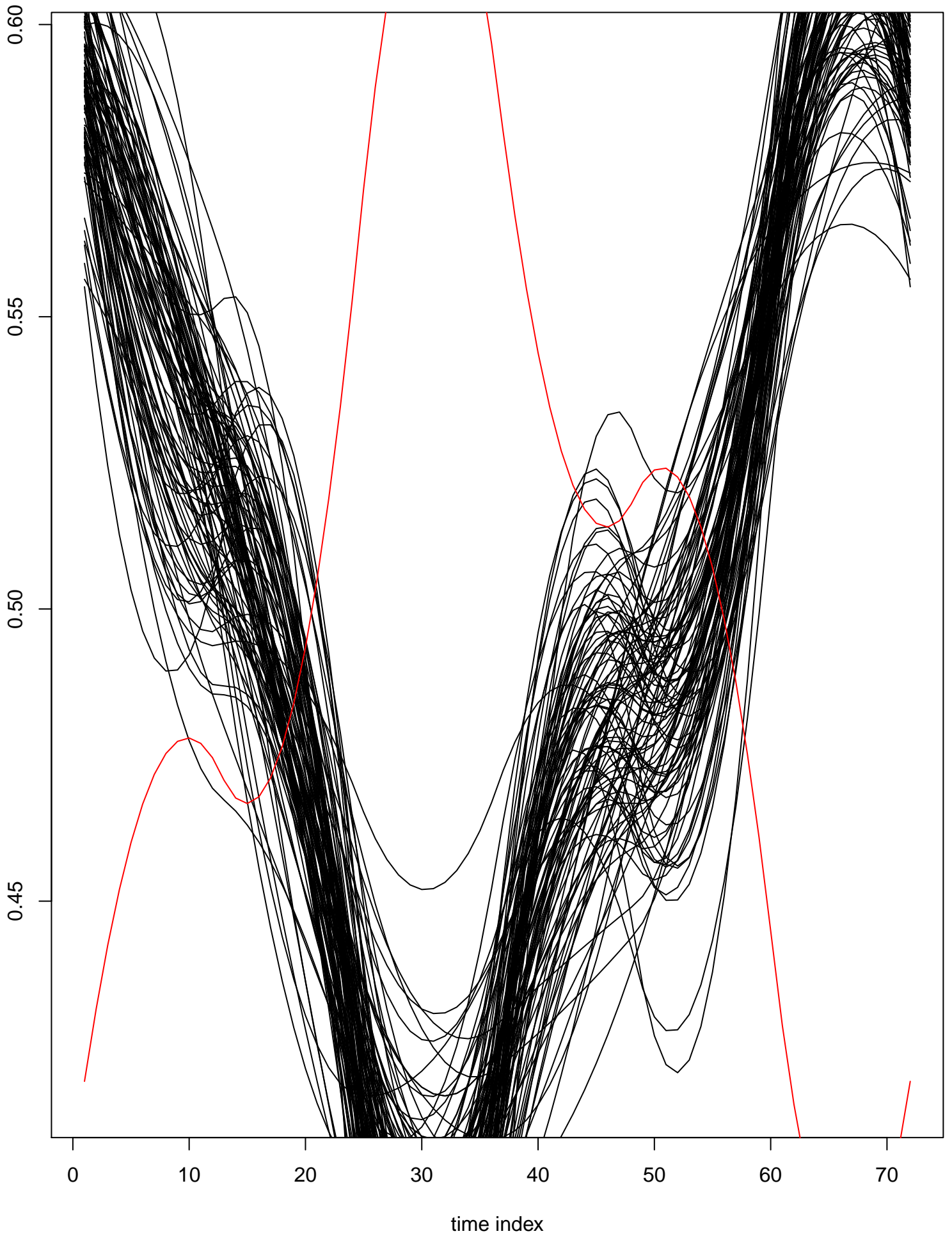
posterior samples of lambda
