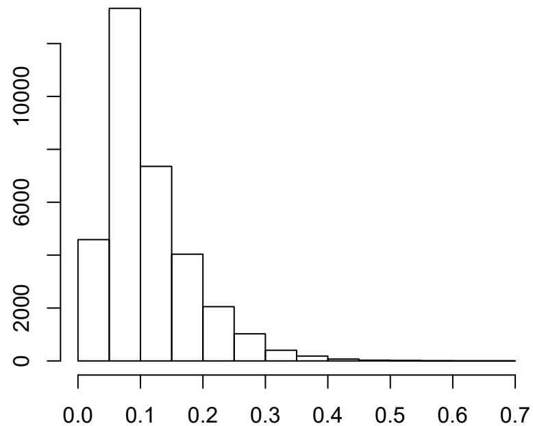
Unconstrained posterior SDs
